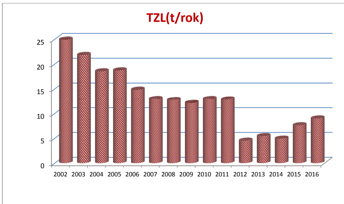
Graf množstva vypustených emisií tuhých znečisťujúcich látok v jednotlivých rokoch.
