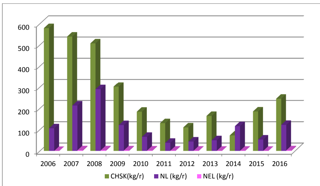
Graf množstva vypustených látok v jednotlivých rokoch do recipientu Vlára
